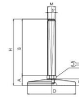
MISE À NIVEAU Pied
