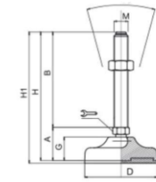
MISE À NIVEAU Pied à rotule
