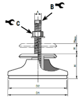
ANTI-VIBRATOIRE Pied statique
